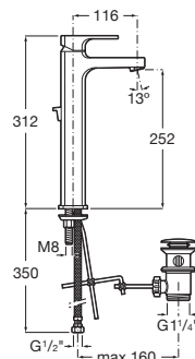
技术图
